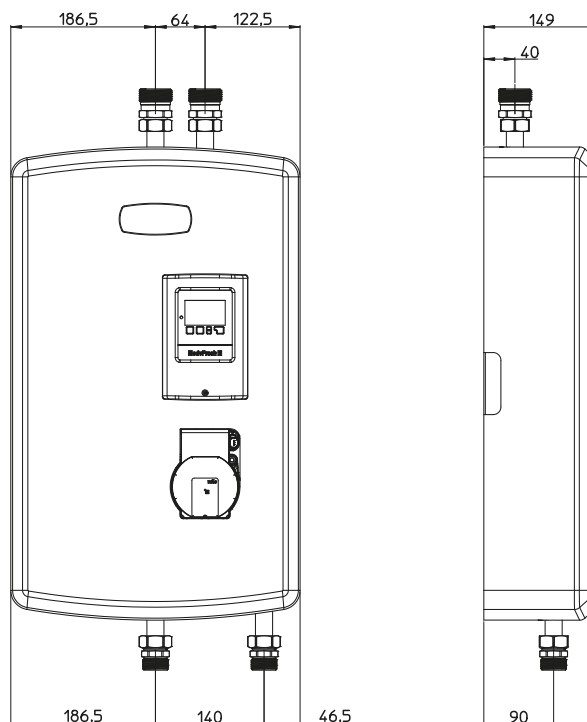
Illustration 3: Encombrements et entraxes significatifs du module
