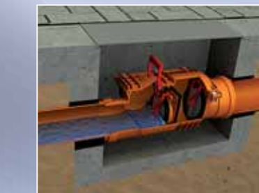
Blockierte Klappe – Doppelrückstauschutz
