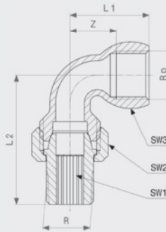
Verschraubung - Rotguss oder Siliziumbronze Modell 3098
