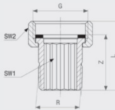
Anschlussverschraubung - Rotguss oder Siliziumbronze Modell 3335
