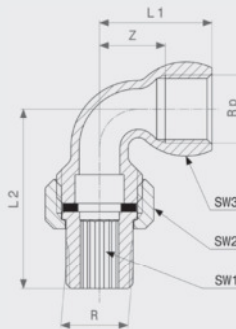
Verschraubung - Rotguss oder Siliziumbronze Modell 3088
