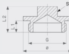
Stopfen - Messing Modell 1751
