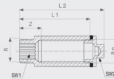
Hahnverlängerung - Rotguss oder Siliziumbronze Modell 3527
