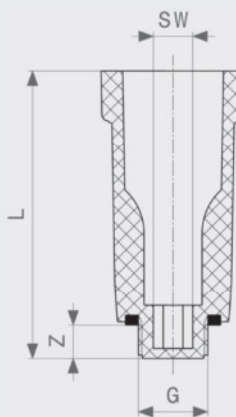
Abdruckstopfen - Kunststoff Modell 1516
