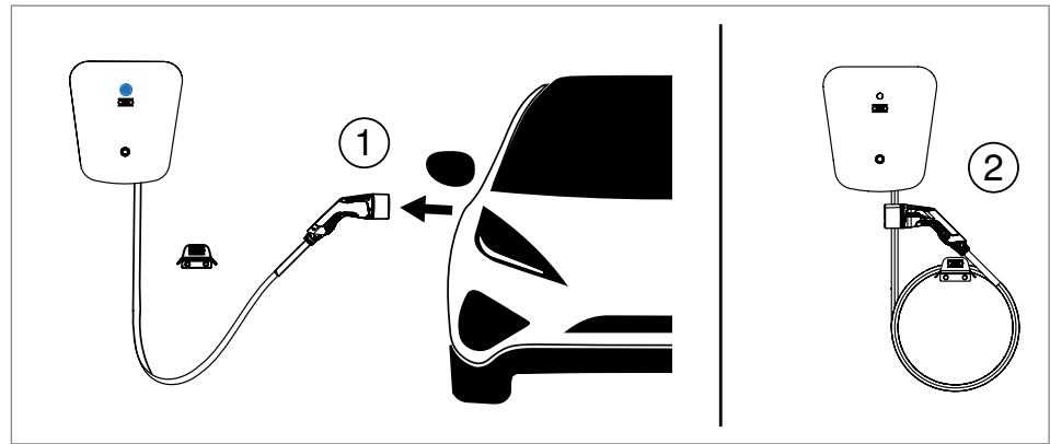
Abb. 11: Ladevorgang beenden
