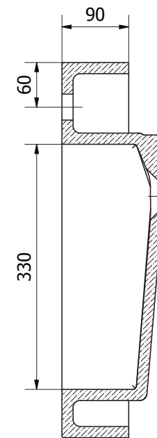
SEZIONE B-B
