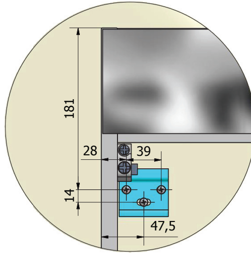
DETTAGLIO B
