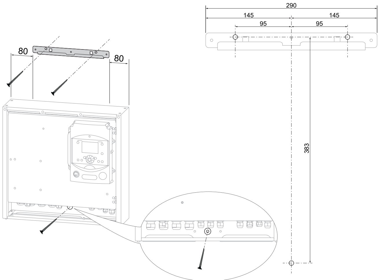
Abb. 4 - Befestigung der Halterung
