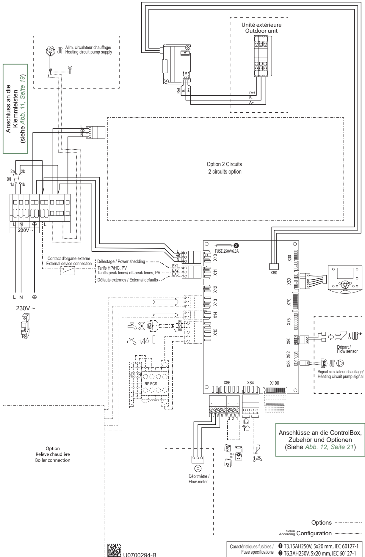
Abb. 20 - Elektrische Verkabelung ControlBox
