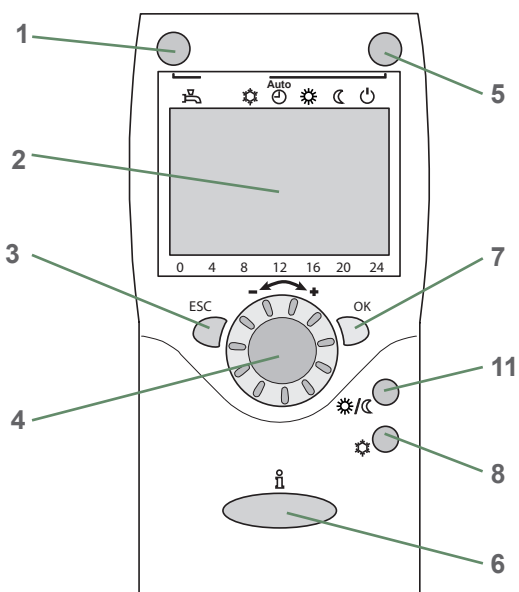
Abb. 13 - Raumtemperurregler T75 / T78
