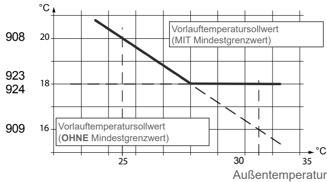
Vorlauftemperatursollwert
