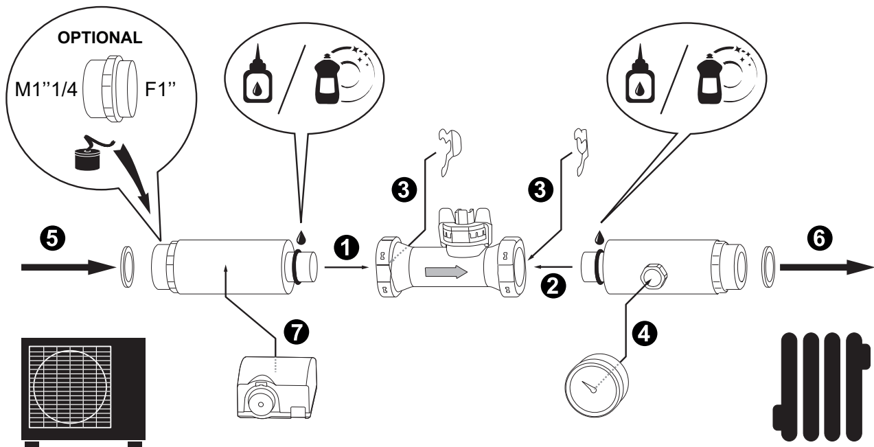
Abb. 6 - Montage der Rohrleitungen und des Durchflussmessers
