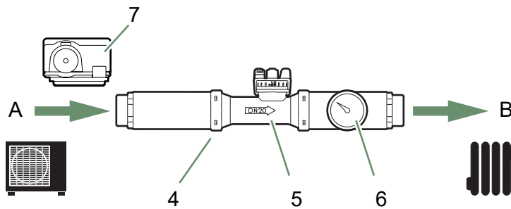
Abb. 2 - Bauteile
