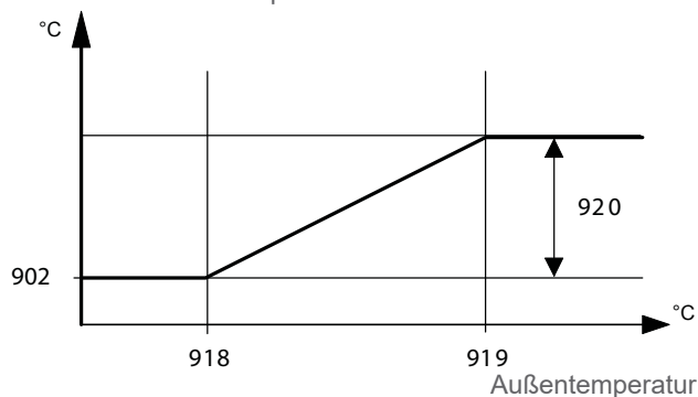
Sollwert Komforttemperatur
