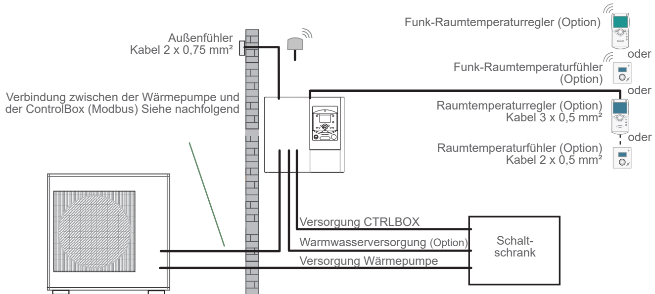
Abb. 7 - Übersicht über die elektrischen Anschlüsse für eine einfache Anlage
