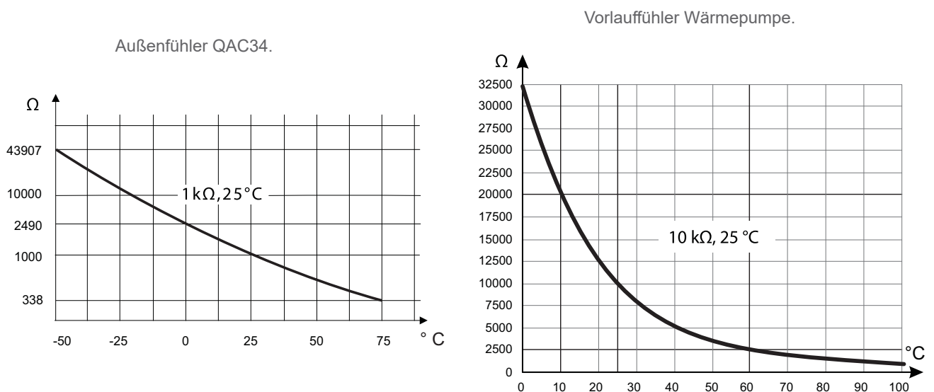
Abb. 3 - Ohmsche Werte der Fühler
