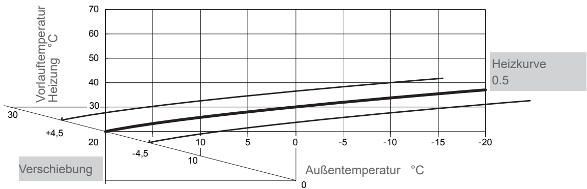
Abb. 18 - Verschiebung der Heizkurve (Zeile 721)
