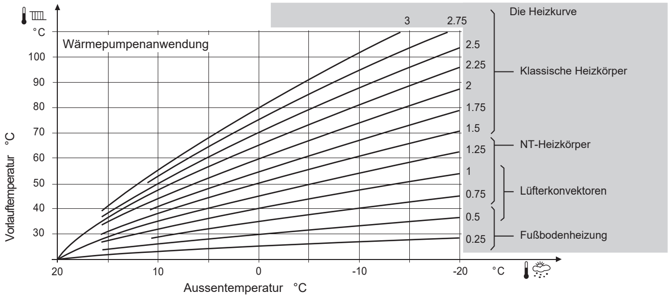
Abb. 17 - Heizkurve (Zeile 720)
