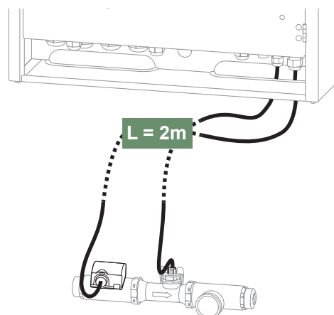
Abb. 9 - Anschluss des Durchflussmessers und des Heizungsvorlauffühlers
