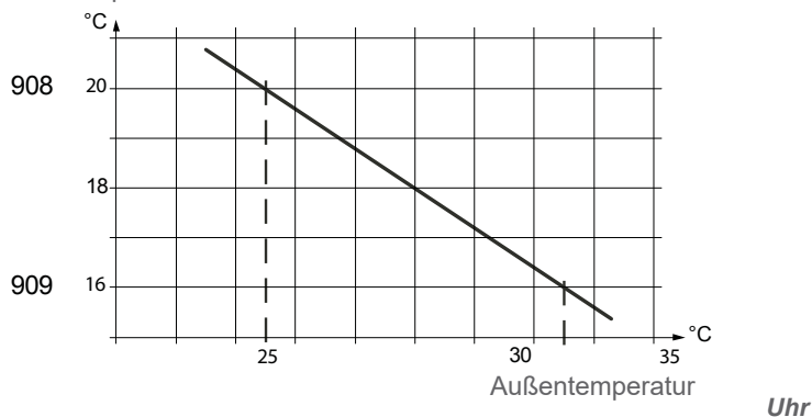
Vorlauftemperatursollwert
