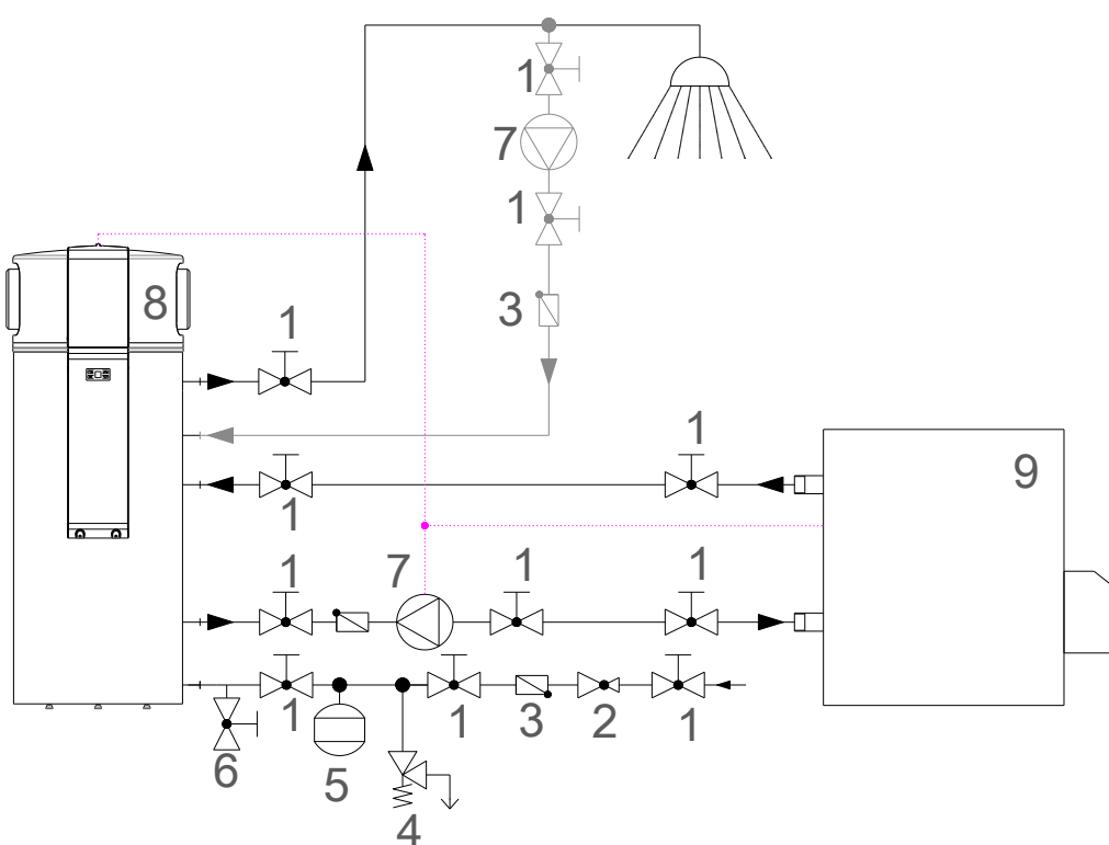
Abbildung 9: Wärmepumpe in Kombination mit Kessel
