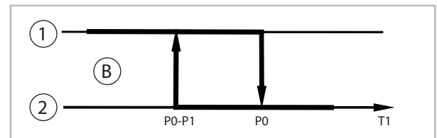
Abb. 17: Kontrolllogik Normal Heizen
