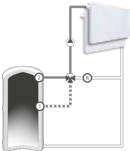
Réservoir de stockage, mélange
