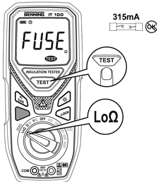
Illustration 12: Contrôler le fusible
