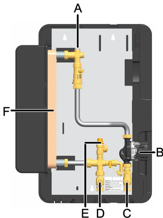
Speicherkreis
