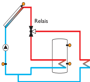
Variante Ventil
