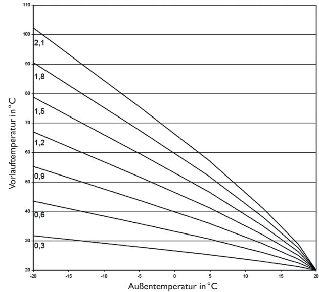
Heizkennlinien
