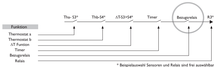
Bezugsrelais
