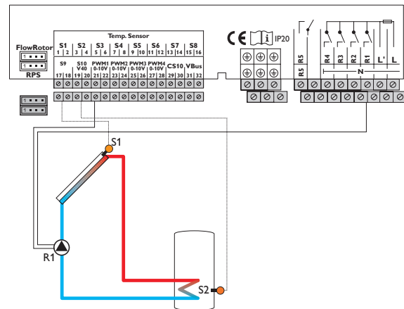
Beispiel für den elektrischen Anschluss einer Hocheffizienzpumpe
