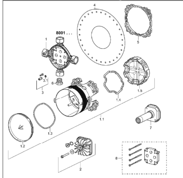
Produktzeichnung
