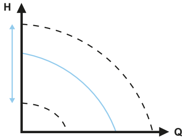
Abb. 26 Konstantkennlinien-Einstellungen
