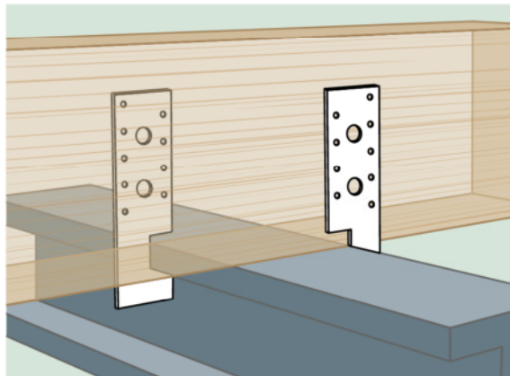
Anwendungsbeispiel SXHE an Stahlträger
