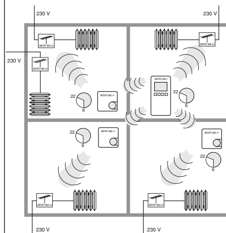
Bild 3: Zeitsteuerung mit Master- und Slaveregler
