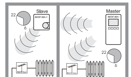
Bild 2: Einfache Master/Slave Funktion
