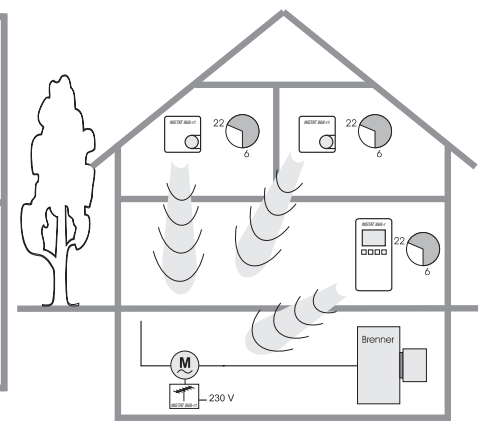
Bild 4: Pumpenlogik mit Master und Slaves
