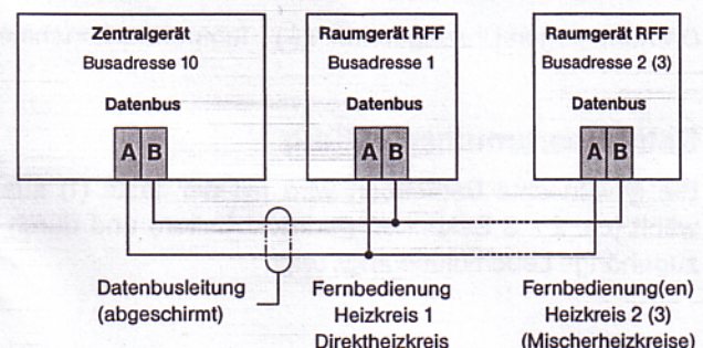
Abb.3 Datenbusführung
