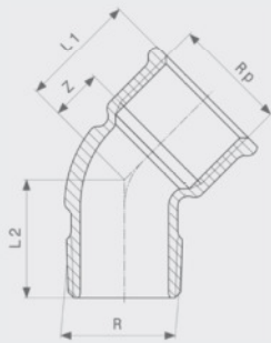
Bogen 45° - Rotguss oder Siliziumbronze Modell 3121
