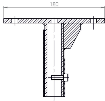
PRZEKRÓJ A-A SKALA 1:2
