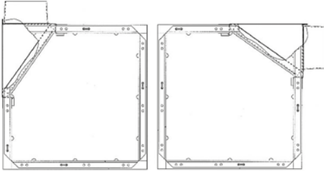
Einbaulage 10.00 Uhr
