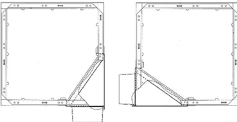
Einbaulage 04.00 Uhr
