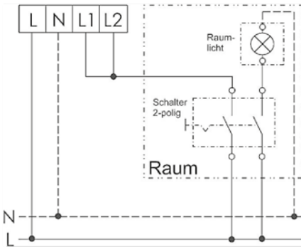
Einstufiger Betrieb
