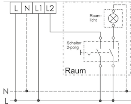
Zweistufiger Betrieb
