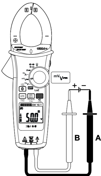
Bild 2: Gleichspannungsmessung Fig. 2: Direct voltage measurement Fig. 2: Mesure de tension continue Fig. 2: Meten van gelijkspanning
