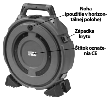
Obrázok 1B – Zariadenie na čistenie odtokov RIDGID® FlexShaft
