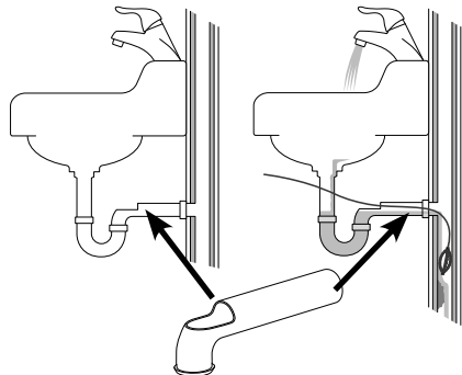
Slika 3 - Montaža stenske cevi
