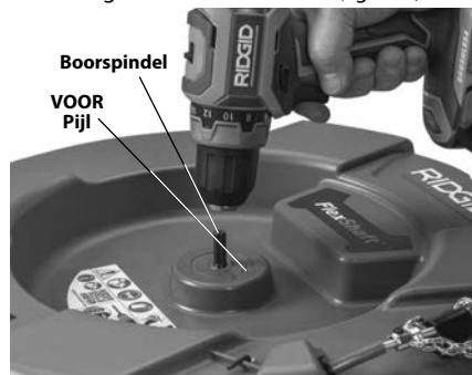
Figuur 4 – De boormachine aan de boorspindel bevestigen
