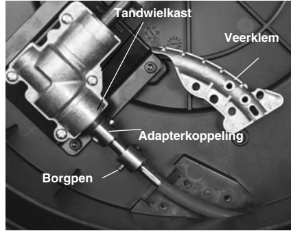
Figuur 15 – Geopende behuizing van de afvoerstopper
