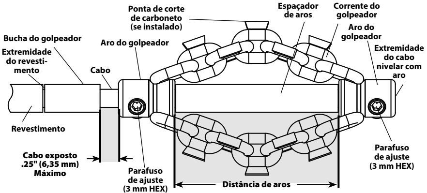
Figura 10 – Instalação/Ajuste do golpeador com corrente
