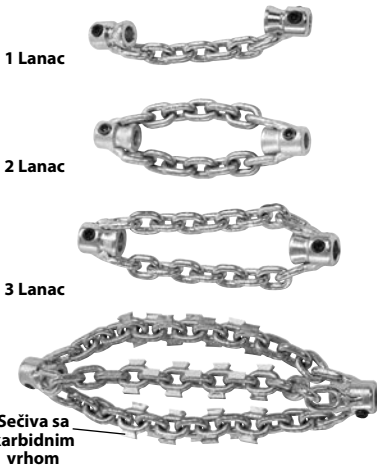
Slika 8 – Lančani udarači
