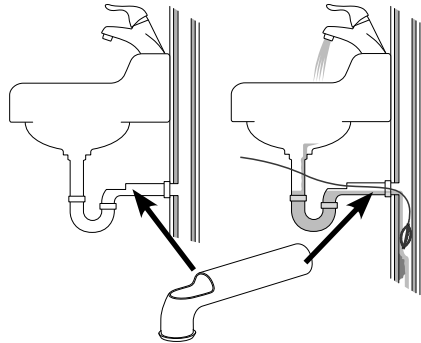
Figuur 3 – Wandbuisinstallatie
