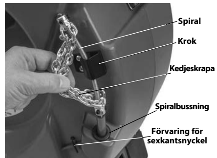
Figur 1C – Spiralände/kedjeskrapa
