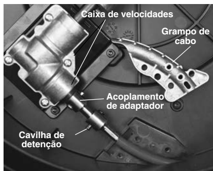
Figura 15 – Alojamento da máquina de limpeza de tubagens aberto
