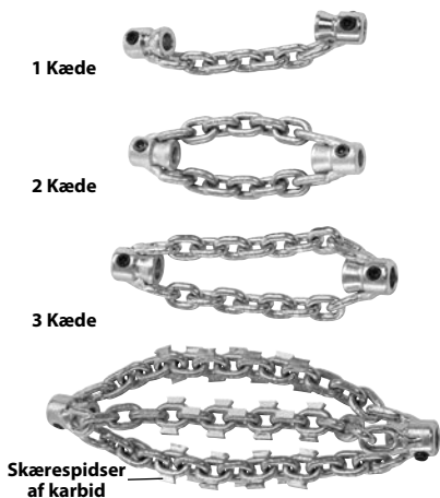
Figur 8 – Kædeskrabere
