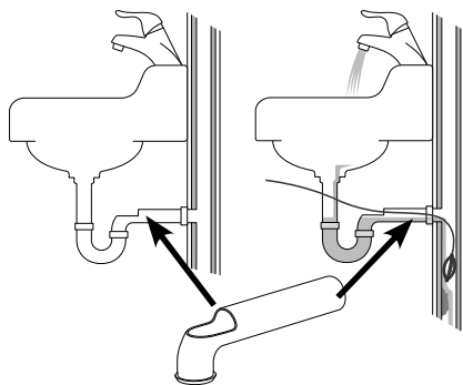
Slika 3 – Instalacija zidne cevi
