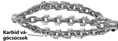
8. ábra – Láncos fejek
