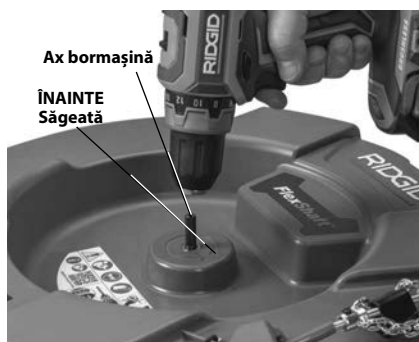
Figura 4 – fixarea bormașinii pe axul acesteia
