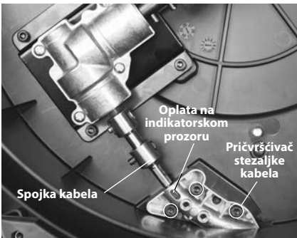
Slika 16 – Zamjena sklopa kabela
