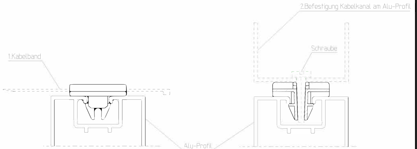
Einbaudarstellung 1:1
