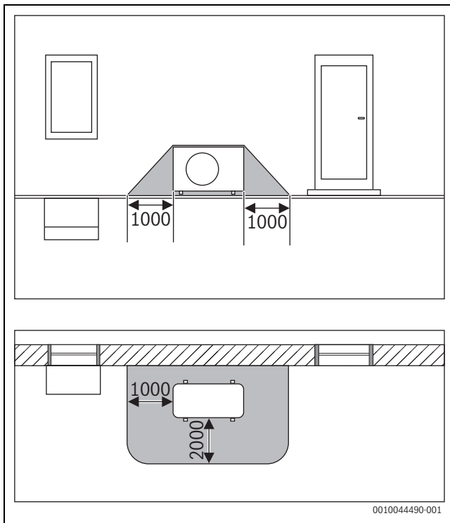
Сл. 43 Заштитено подрачје, подна надворешна единица на ѕид (димензии во mm)
