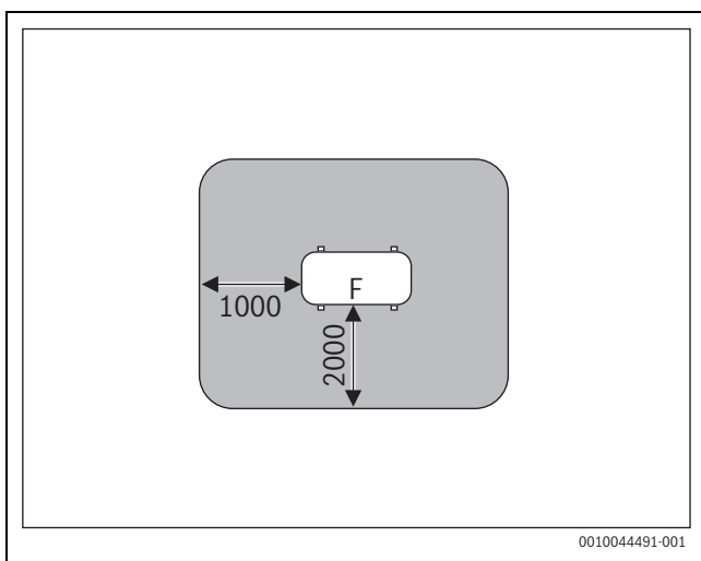
Pav. 38 Apsaugos zonos matmenys (mm), kai išorinis blokas stovi ant žemės arba ant stogo
