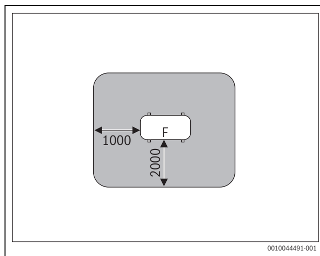
Fig. 26 Volume de protection pour la mise en place au sol sur le terrain ou le toit (dimensions en mm)
