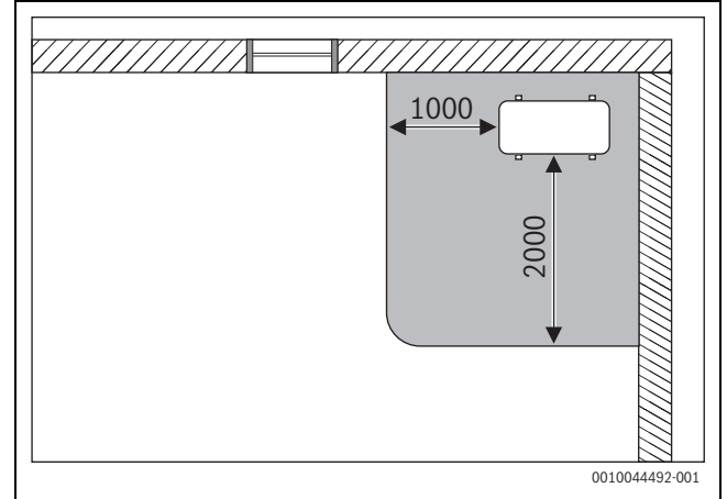
fig. 66 Zona e mbrojtjes, njësi e jashtme me qëndrim në dysHEME në një kënd (përmasat në mm)
