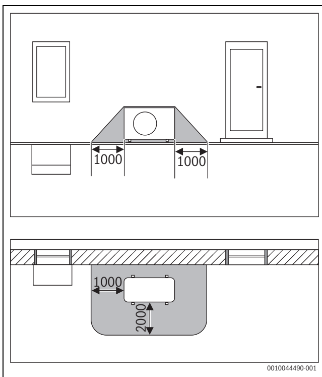
Fig. 19 Sector de protección, unidad exterior sobre el suelo junto a una pared (medidas en mm)
