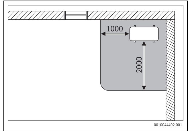
Res. 72 Koruma bölgesi, bir köşeye yaslanmış ayaklı dış ünite (ölçüler mm olarak verilmiştir)
