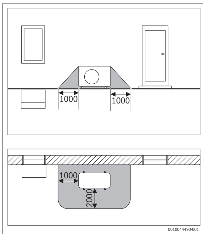
Σχ. 13 Προστατευμένη περιοχή, εξωτερική μονάδα τοποθετημένη στο δάπεδο σε τοίχο (διάσταση σε mm)
