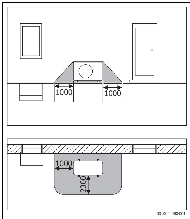
Fig. 7 Schutzbereich, bodenstehende Außeneinheit an einer Wand (Maße in mm)
