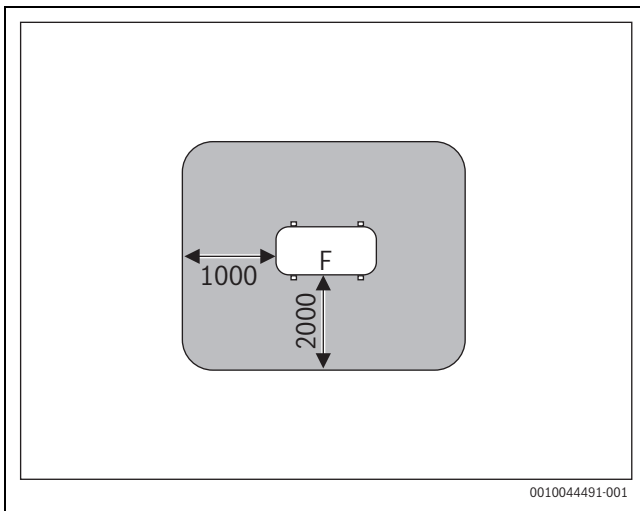
Res. 71 Dış ünitenin arazi veya tavan zemin üzerine yerleştirilmesi durumunda koruma bölgesi (ölçüler mm olarak verilmiştir)
