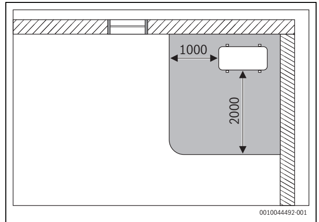
Joon. 24 Ohupiirkond, nurgas põrandal seisev välisseade (mõõdud mm-tes)
