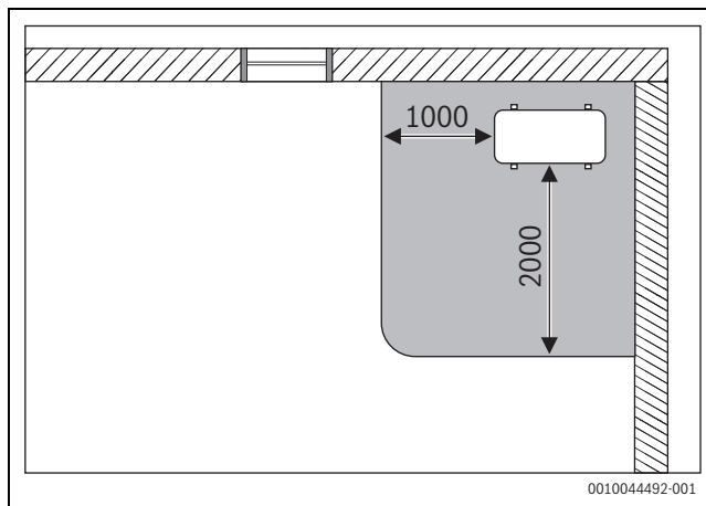
Σχ. 15 Προστατευμένη περιοχή, εξωτερική μονάδα τοποθετημένη στο δάπεδο σε γωνία (διάσταση σε mm)
