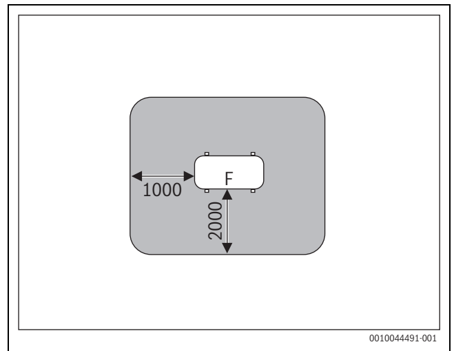
Сл. 44 Заштитено подрачје при инсталација на под на имот или покрив (димензии во mm)
