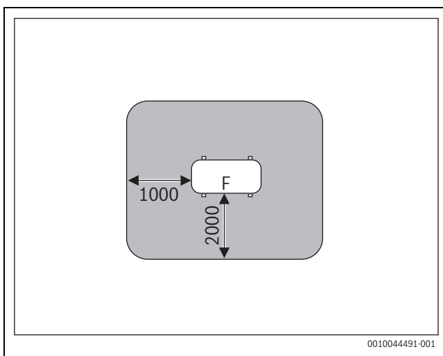
Att. 41 Aizsardzības zona, uzstādot iekārtu uz zemes uz gruntsgabala vai jumta (izmēri mm)
