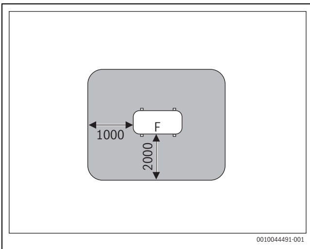
Joon. 23 Ohupiirkond paigaldusel kinnistul maapinnale või katusele (mõõdud mm-tes)
