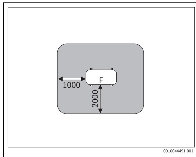
Fig. 56 Zonă de protecție la amplasarea pe podea, pe teren sau pe acoperiș (dimensiuni în mm)
