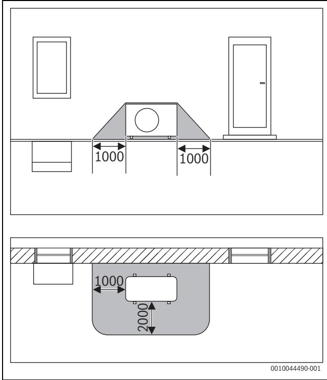
Res. 70 Koruma bölgesi, bir duvara yaslanmış ayaklı dış ünite (ölçüler mm olarak verilmiştir)
