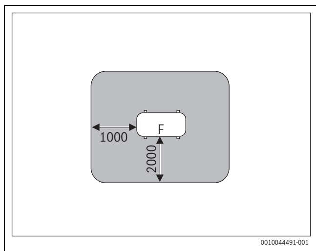
Fig. 8 Schutzbereich bei Aufstellung auf dem Boden auf dem Grundstück oder Dach (Maße in mm)
