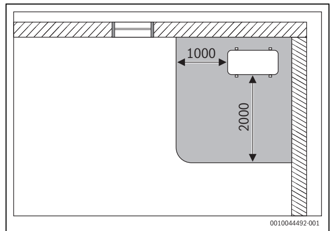
Fig. 21 Sector de protección, unidad exterior sobre el suelo en una esquina (medidas en mm)
