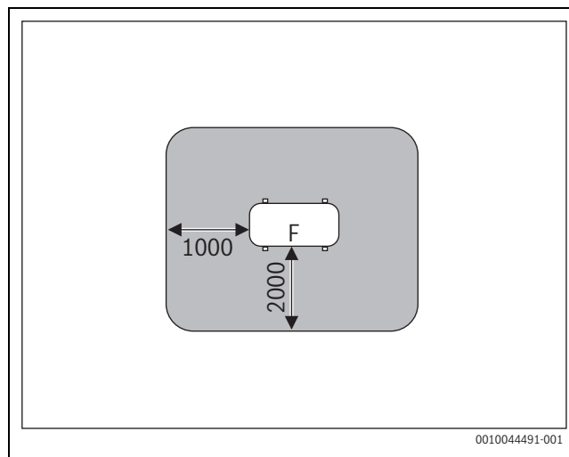
Rys. 50 Strefa ochronna dla urządzenia ustawionego na gruncie na parceli lub na dachu (wymiar w mm)
