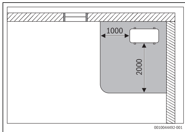
Fig. 9 Schutzbereich, bodenstehende Außeneinheit in einer Ecke (Maße in mm)
