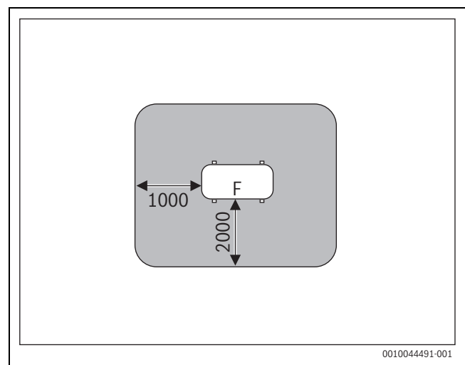
32. ábra Védett terület az ingatlanon a padlón vagy a tetőn felállítva (méretetek mm-ben)
