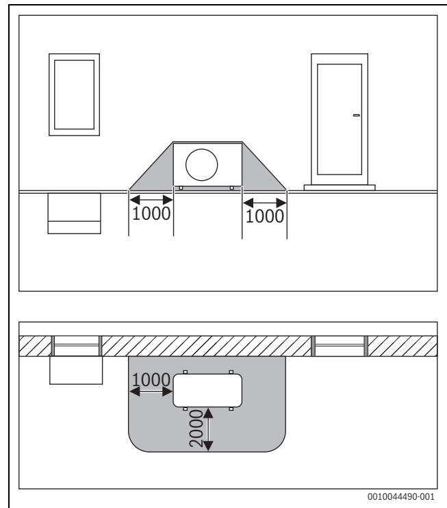
31. ábra Védett terület, padlón álló kültéri egység a falnál (méretetek mm-ben)
