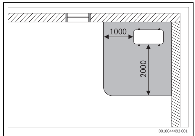
Сл. 45 Заштитено подрачје, подна надворешна единица во агол (димензии во mm)
