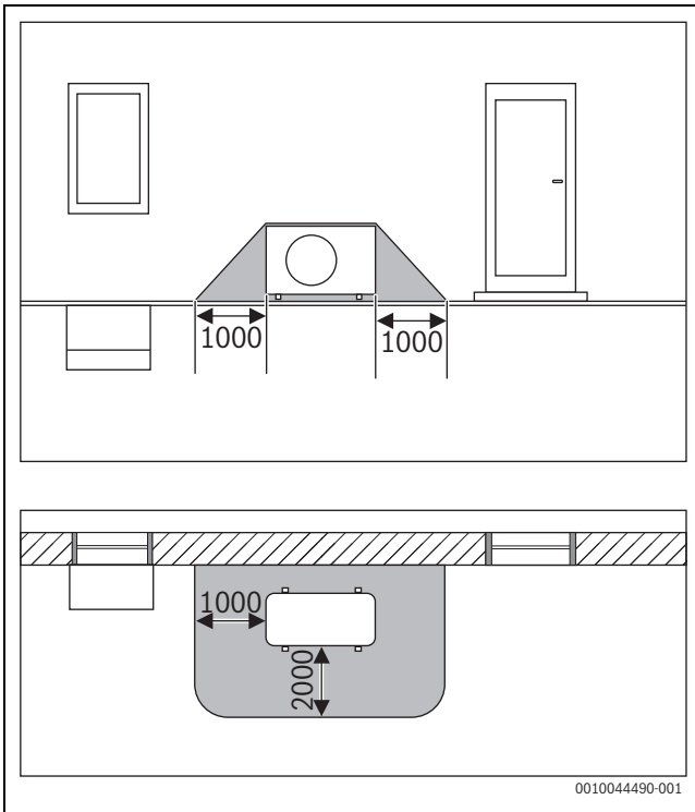
Joon. 22 Ohupiirkond, seina ääres põrandal seisev välisseade (mõõdud mm-tes)
