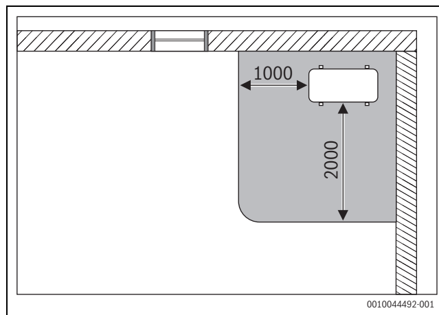
Sl. 63 Varnostno območje, talna zunanja enota v kotu (mere v mm)
