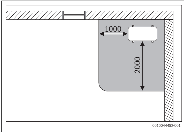
Rys. 51 Strefa ochronna, jednostka zewnętrzna posadowiona na gruncie w narożniku (wymiar w mm)
