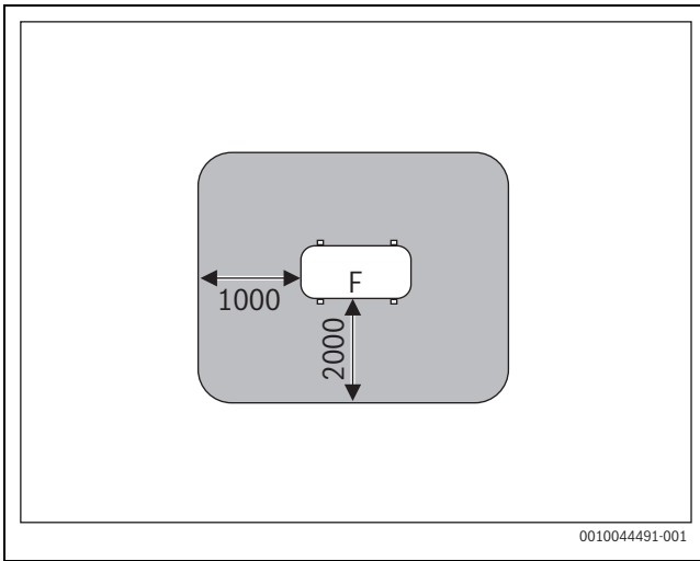
fig. 65 Zona e mbrojtjes kur vendoset përtokë në objekt apo në çati (përmasat në mm)
