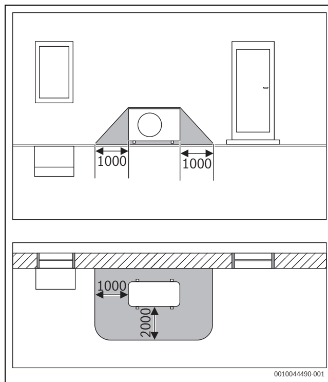
Rys. 49 Strefa ochronna, jednostka zewnętrzna posadowiona na gruncie przy ścianie (wymiar w mm)
