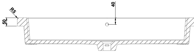
SEZIONE B-B
