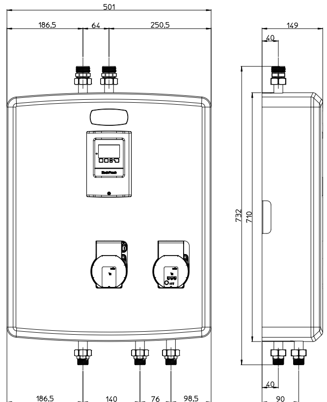
Abb. 3: Abmessungen und Achsabstände
