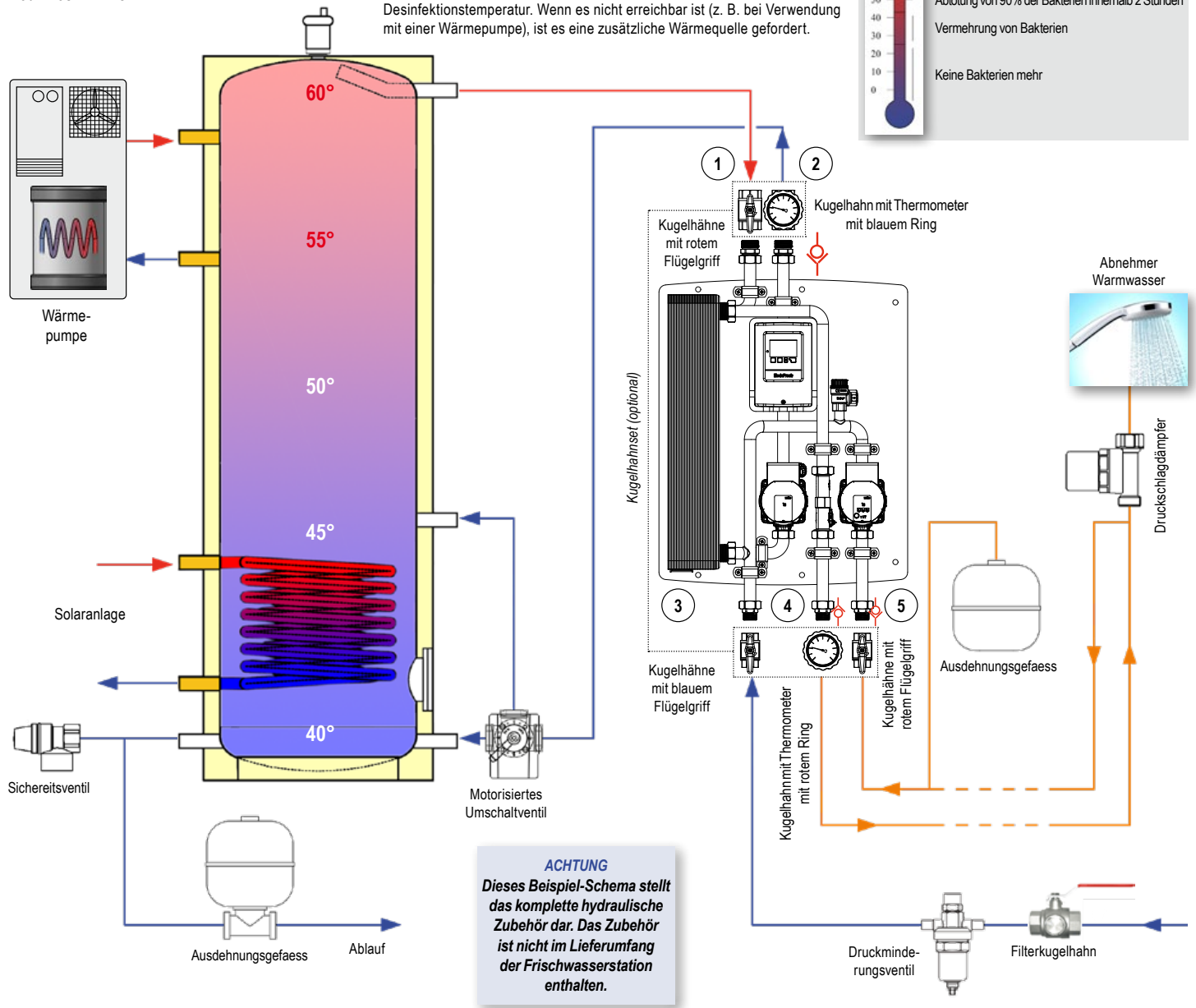
Abb.1: Anlagenschema der Frischwasserstation ModvFresh 2 PDC
