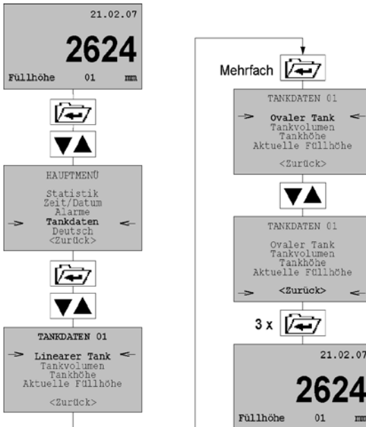
Bild 11: Tankform ändern
