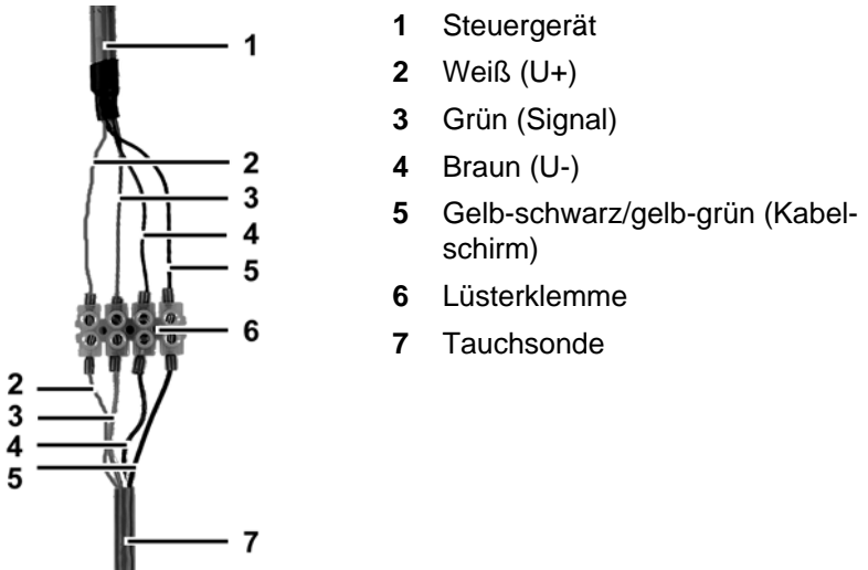
Bild 5: Kabelverbindung Steuerg r t und Tauchsonde
