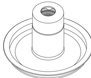
Abb. 28 Spaltrohrtopf mit Lageraufnahme und Keramiklager
