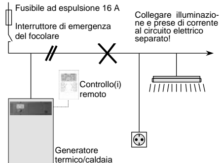
Fig. 3: Instradamento dei cavi elettrici nel focolare
