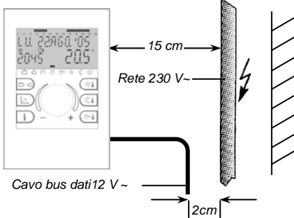
Fig. 1: Distanze minime per installazione elettrica
