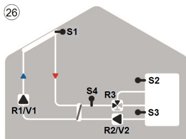
Solar mit Wärmetaucher, 2-Zonenspeicher und Ventil
