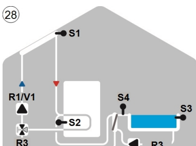
Solar mit Pool, Speicher und Wärmetaucher
