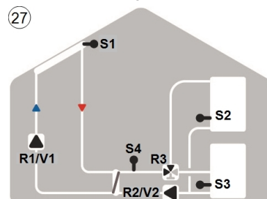
Solar mit Wärmetaucher, 2 Speichern und Ventil
