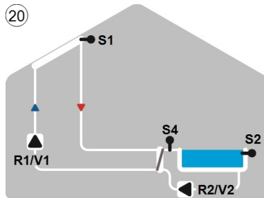
Solar mit Pool und Wärmetaucher
