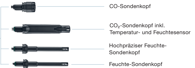
Feuchte-Sondenkopf
