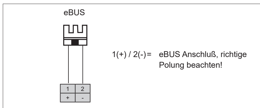
Abb. 4.5 Klemmenblockbelegung Wandsockel
