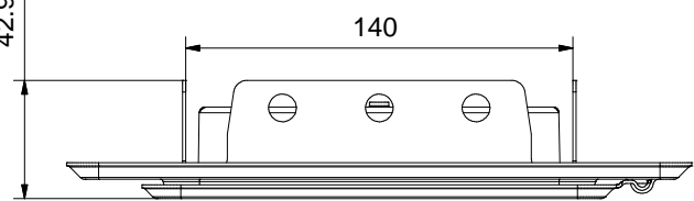
G-G (1:2)
