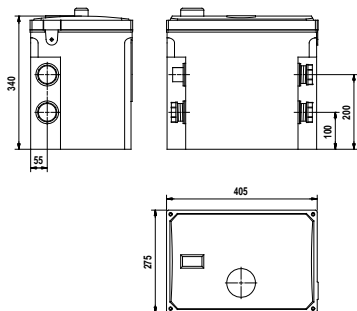
Abb. 2 Maßzeichnungen
