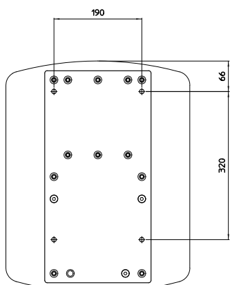
III. 2: Plaque spéciale pour l'installation au mur du module
