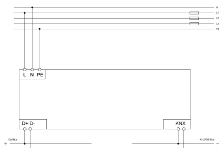
Anschlussbeispiel SCN-DA641.04
