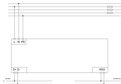
Anschlussbeispiel SCN-DA642.04
