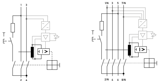
▲ zweipolig (grau: nur Typ B)
