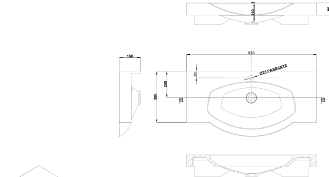
SEZIONE B-B
