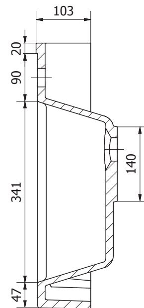
SEZIONE B-B
