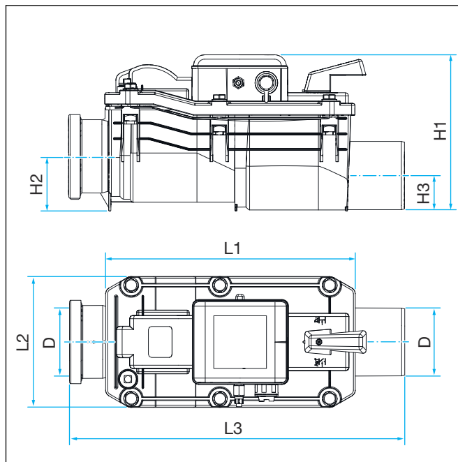
Abb. 7: Einbaumaße
