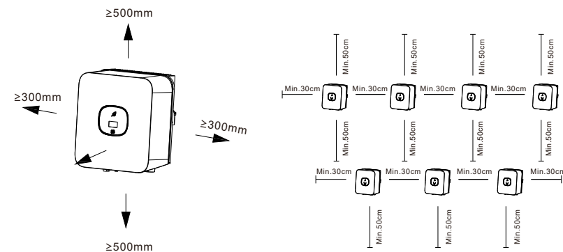
Umgebungsabmessungen eines Wechselrichters
