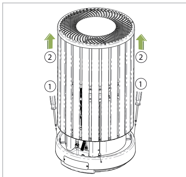
Abb. 3: Demontage des Korbs
