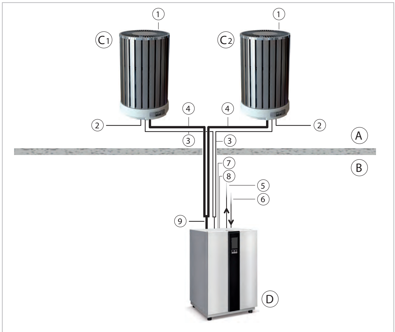
Abb. 2: Systemaufbau HTS 200/260
