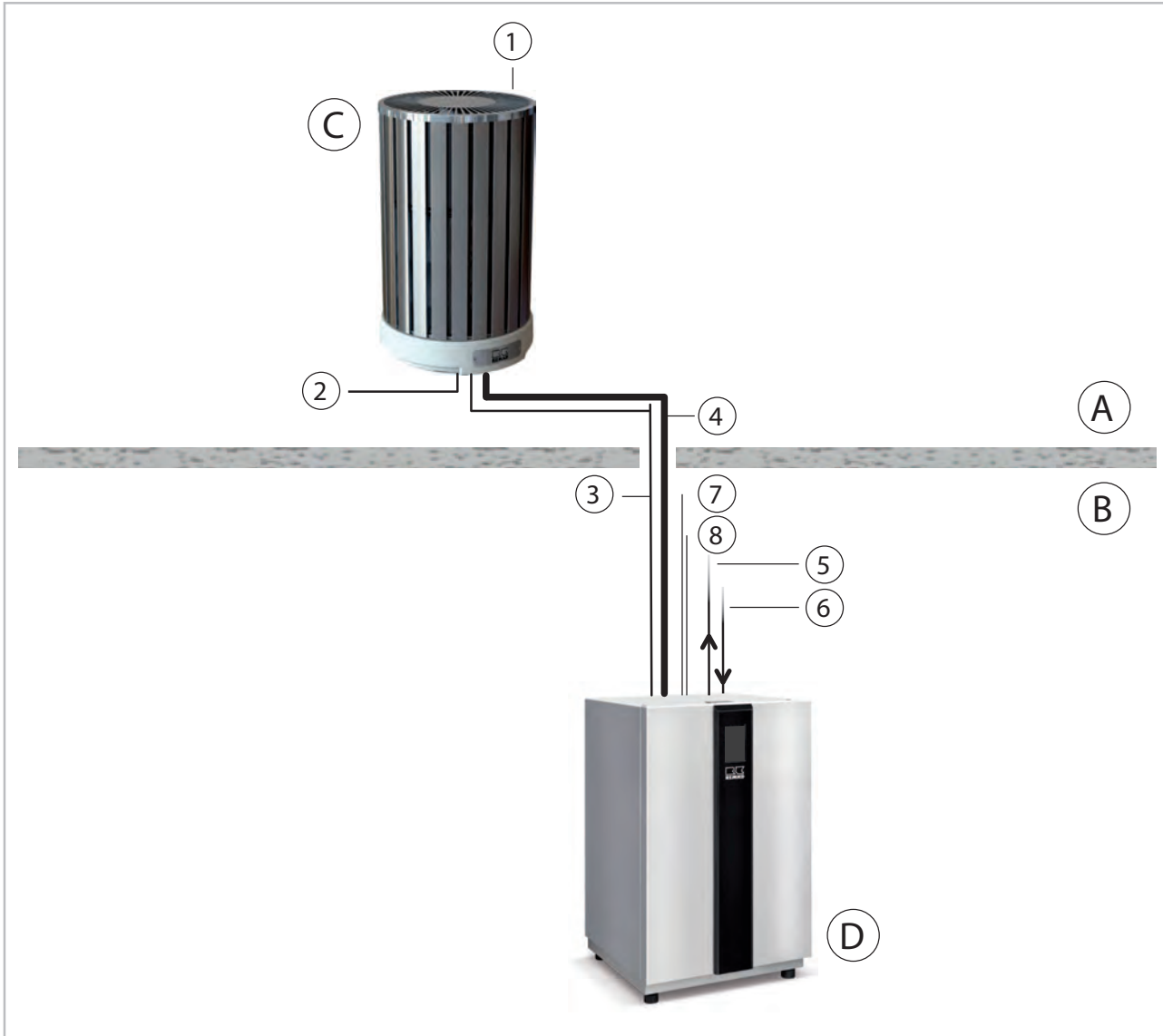
Abb. 1: Systemaufbau HTS 80/90/110/130
