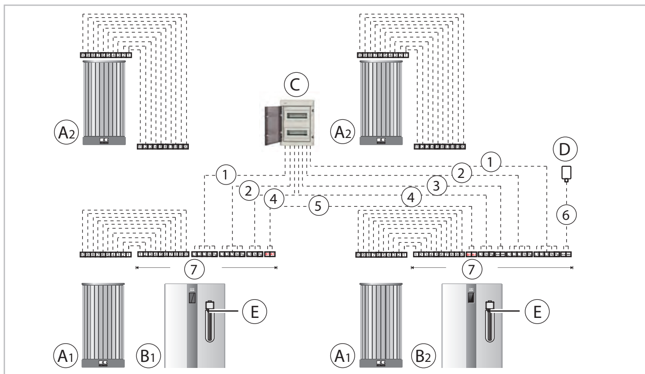
Abb. 21: Klemmbelegung HTS 260 Duo
