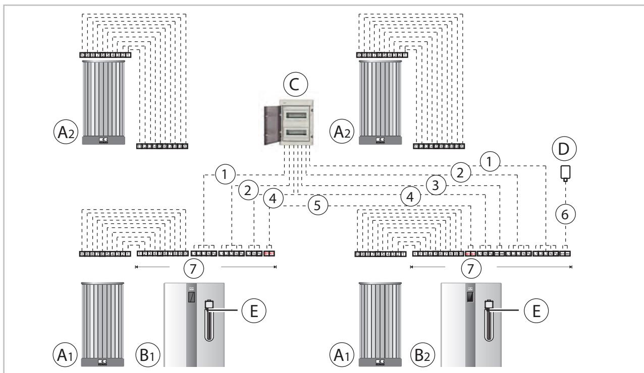
Abb. 19: Klemmbelegung HTS 200 Duo
