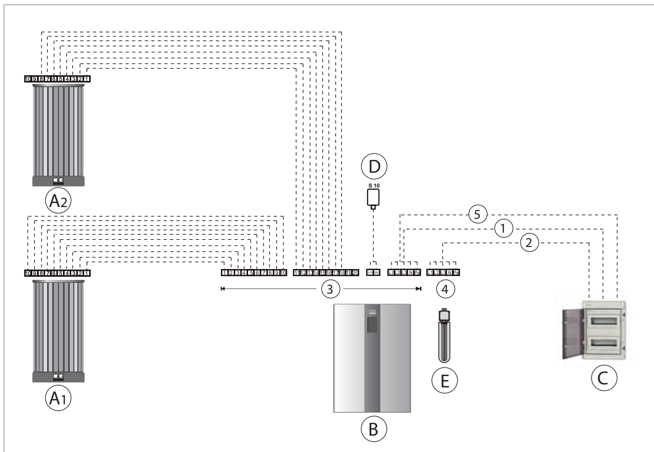
Abb. 17: Klemmbelegung HTS 260
