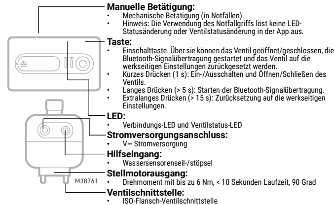
Abb. 2. Komponenten.
