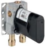
Grundkörper für Unterputz-Thermostat mit Vorabsperung
