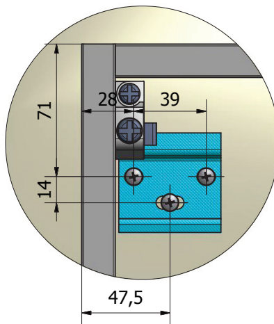
DETTAGLIO A
