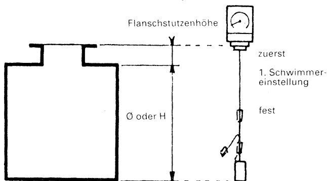
Abb. 1: Instrumenteneinstellung
