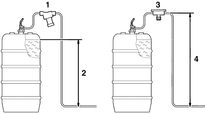
Bild 4: Magnetventil, Membran- oder Kolben-Antiheberventil
