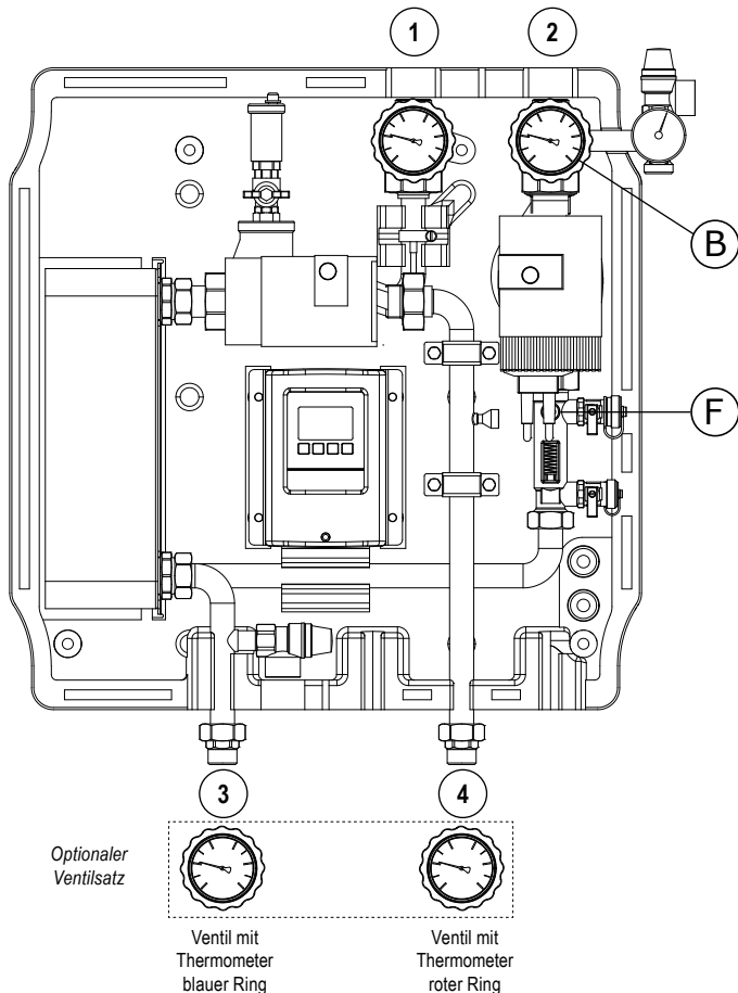
Abb. 1: Schema der Anschlüsse und des optionalen Ventilsatzes
